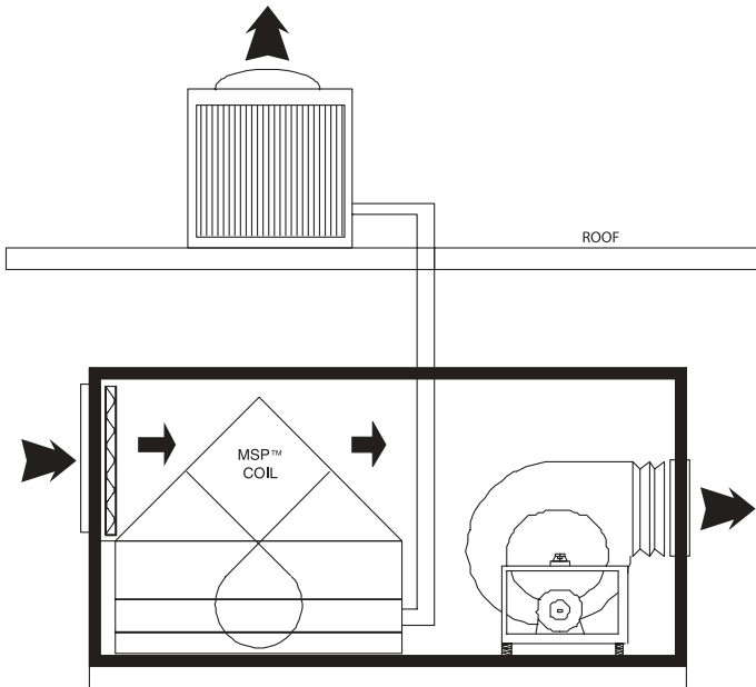
DH Split (Indoor)
